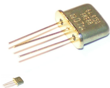
quarz3bein.jpg
